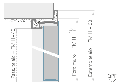
PORTA SENZA BATTUTA INFERIORE - SEZIONE VERTICALE
