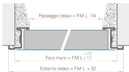
PORTA AD UN'ANTA - SEZIONE ORIZZONTALE
