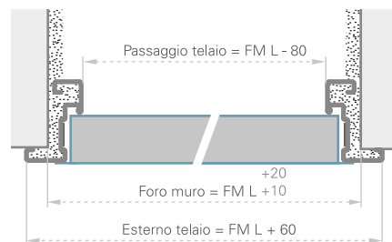
PORTA AD UN'ANTA - SEZIONE ORIZZONTALE
