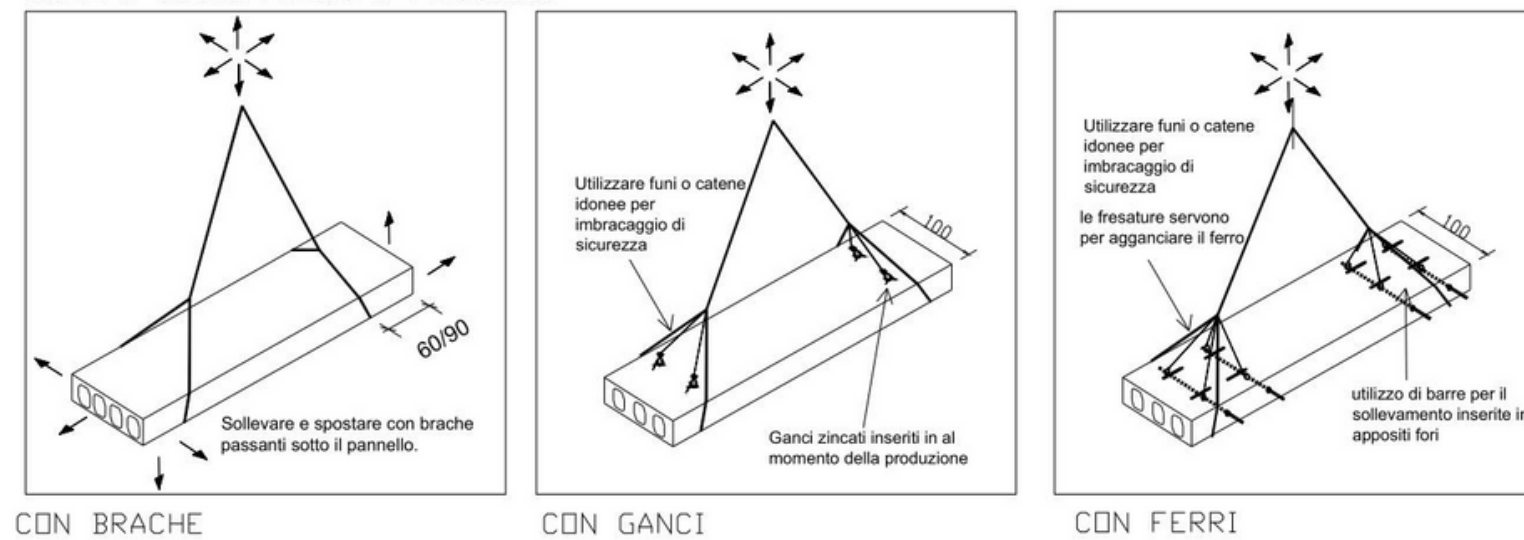
SCHEMI SOLLEVAMENTO PANNELLI
